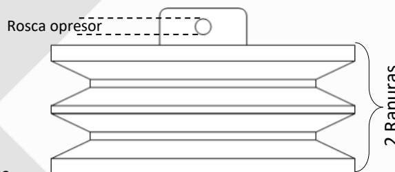
Vista lateral polea
